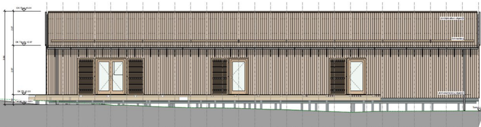
Ansicht West Fassade
