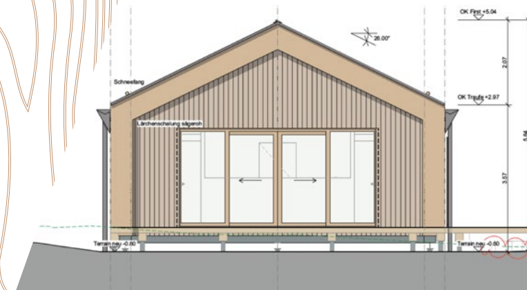
Ansicht Nord Fassade
